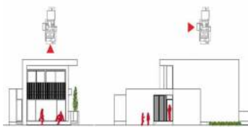
Villa Bonaventura alzados / elevations
